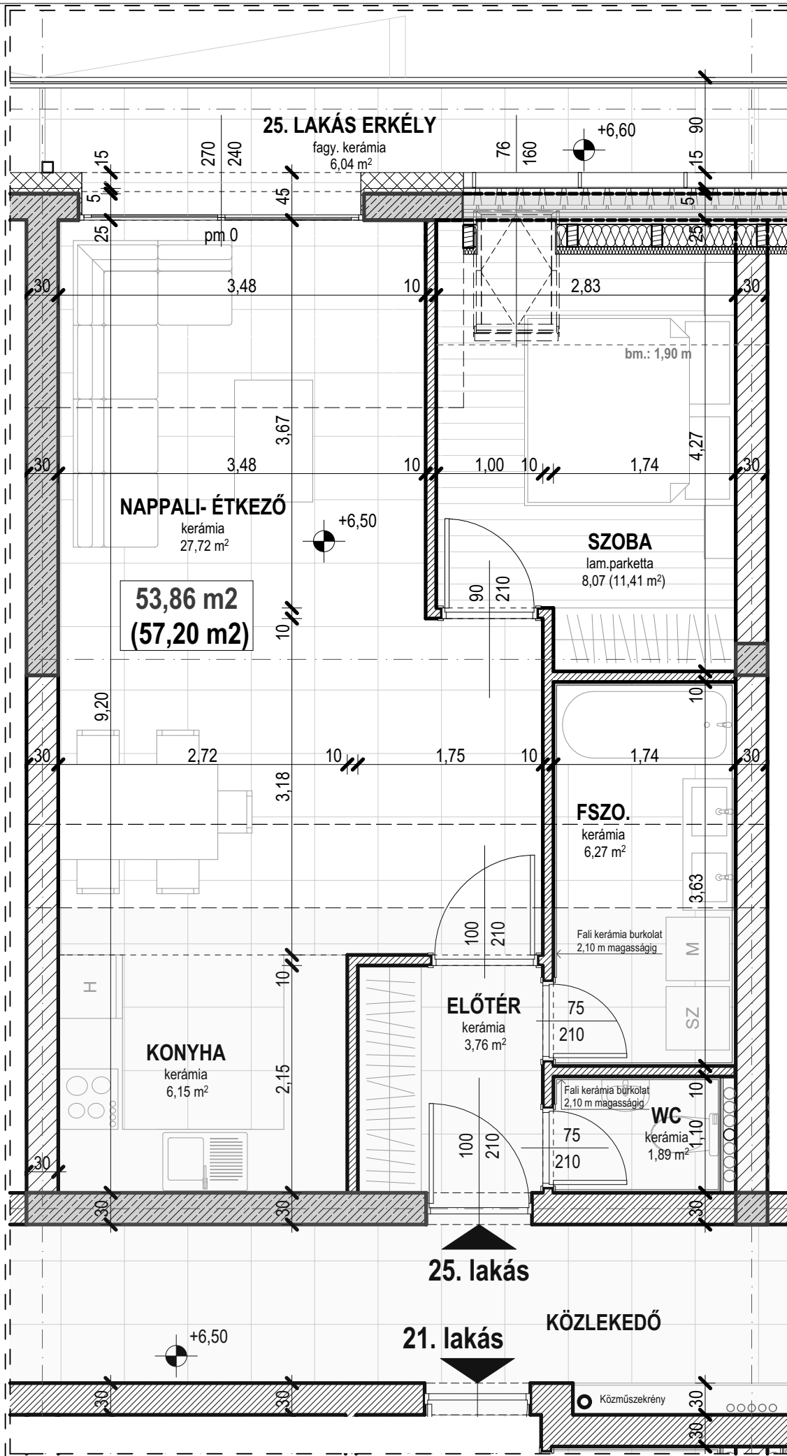
HAJDÚSZOBOSZLÓ, SZURMAI UTCA 4-6. SZ. - TETŐTÉR - 25. LAKÁS - 53,86 m 2 (57,20 m 2 )
